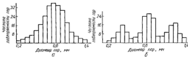
Рис. 8.18. Характер распределения пор по диаметрам в ячеистых материалах: а — одномодальное; б — трехмодальное
