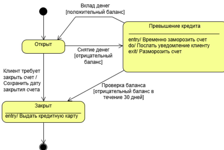
Рисунок 3.9 – Диаграммы активности
