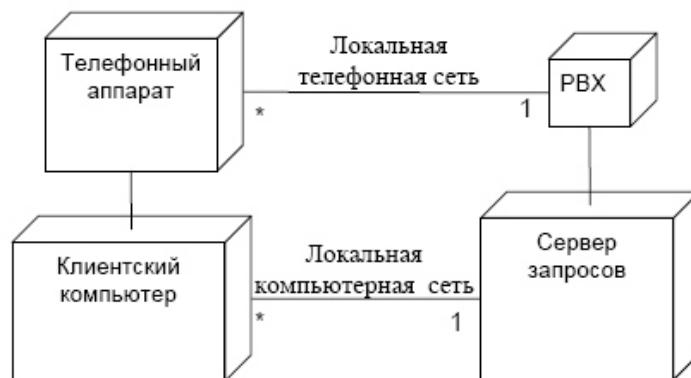
Рисунок 3.7 – Диаграмма развертывания
