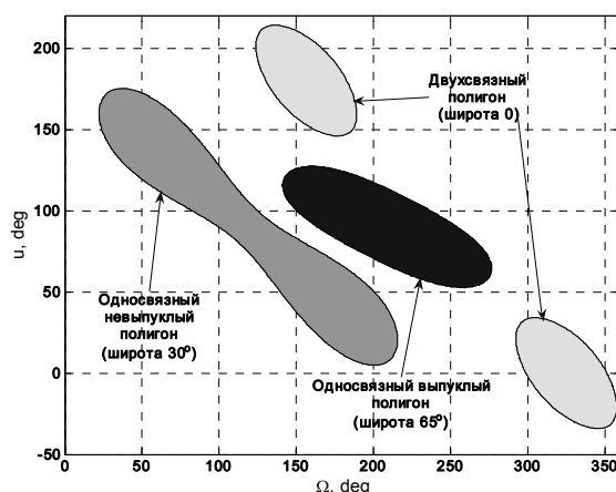
Рис. 5. Примеры полигонов для простейшего обзора (круговая орбита h = 1400\text{км} , i = 52^\circ , \varepsilon = 10^\circ )
