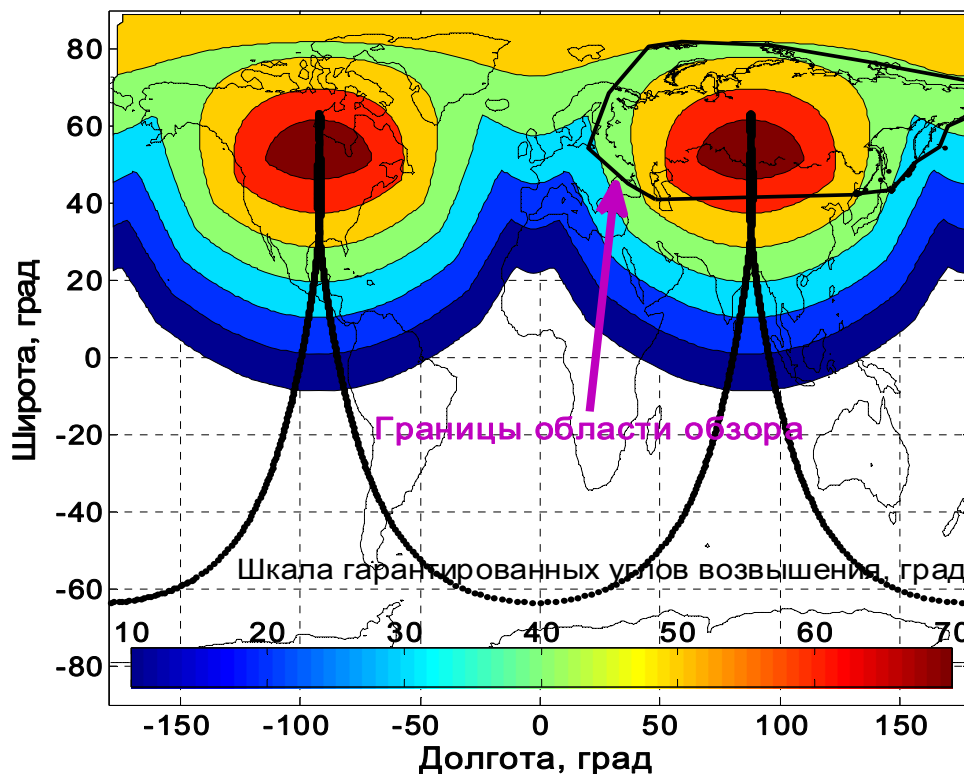
Рис. 18 Характеристики обзора односпутниковой СС на орбите МОЛНИЯ
