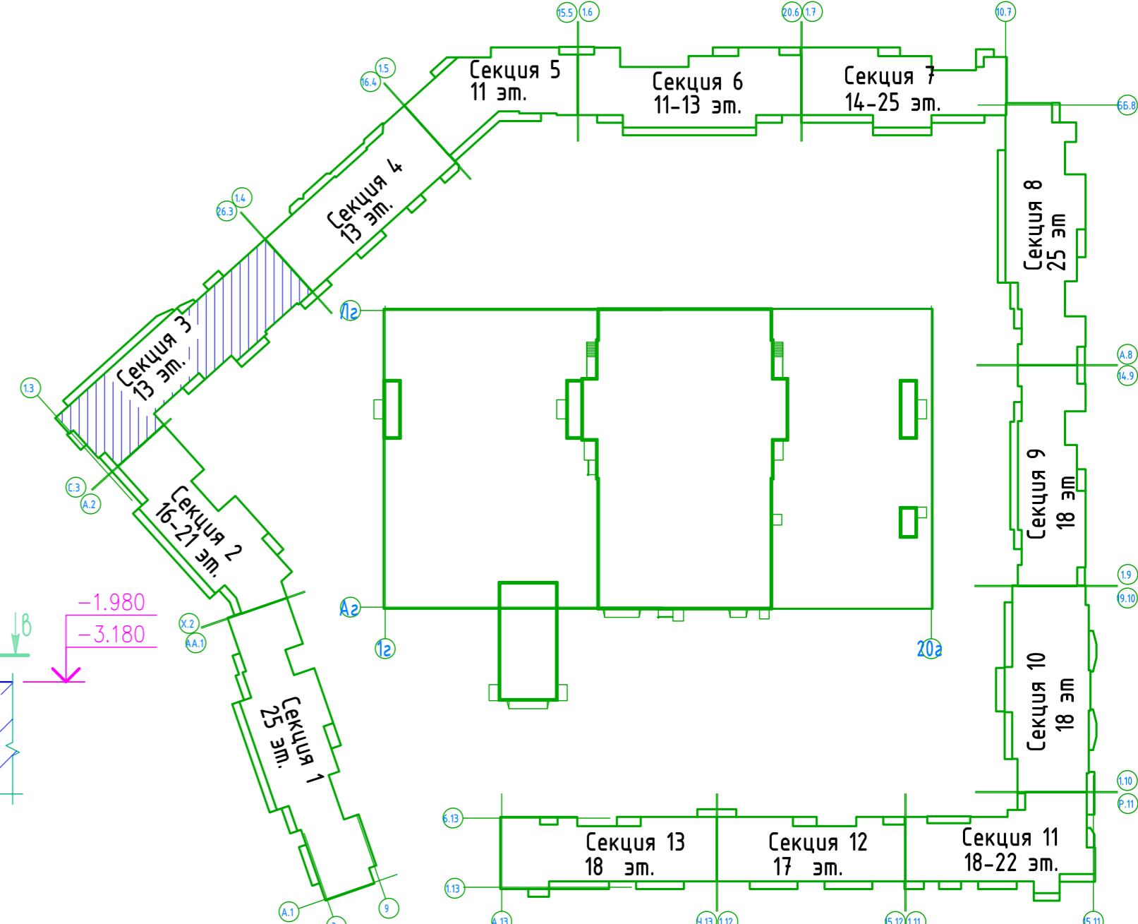
Схема корпуса
